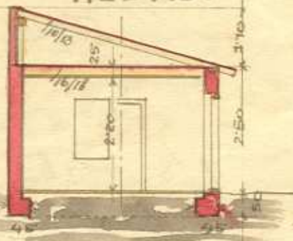
ŘEZ A-B.
