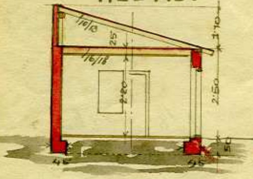
ŘEZ AB.
