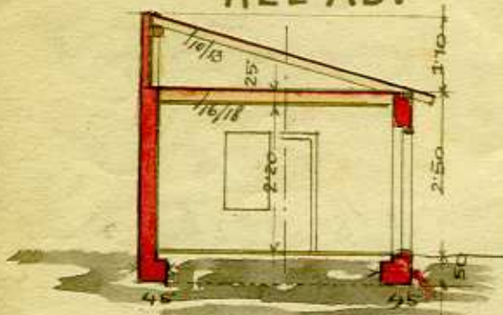
ŘEZ AB.
