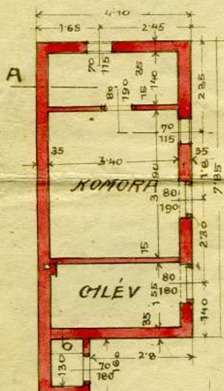
PŘÍZEMÍ.
