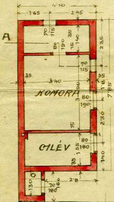
PRÍZEMÍ.
